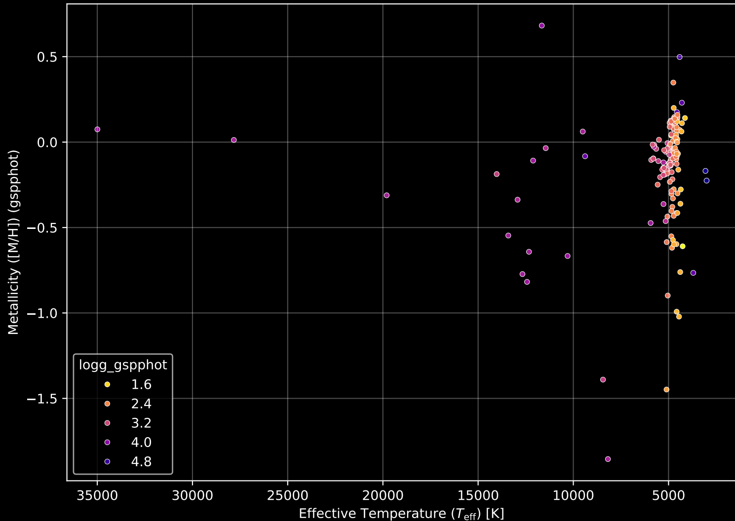
APOGEE DR17 Field: [105-06] Stellar Population Parameters (n= 158)
